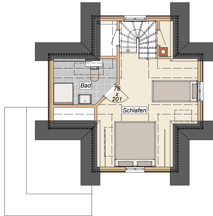
DG: Wohnfläche 16,16 m 2
