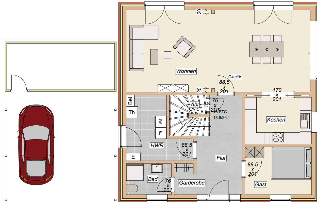
EG: Wohnfläche 85,38 m 2
